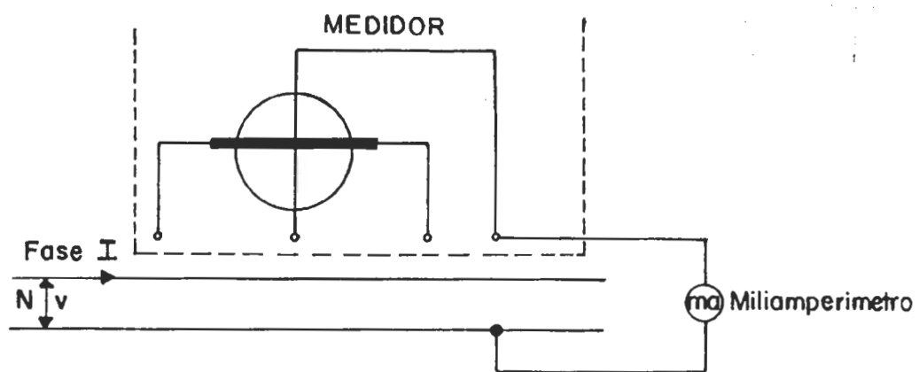
Figura 2. Pérdidas aparentes (en el circuito de voltaje)
