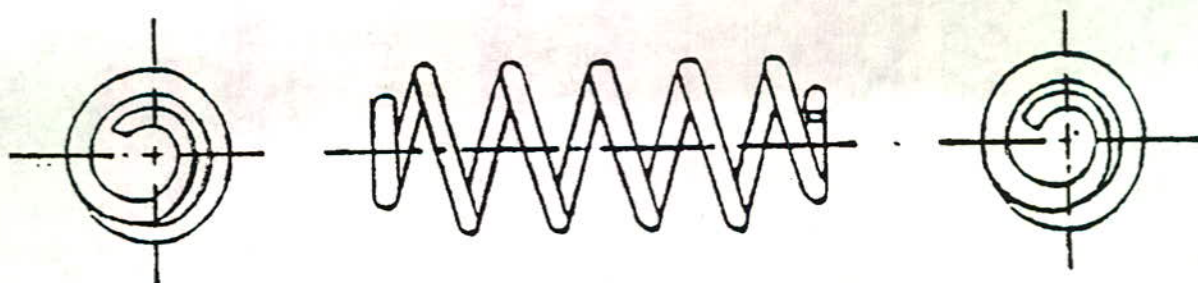
Figura 3c. Dos terminales "Rabo de Cochino"
