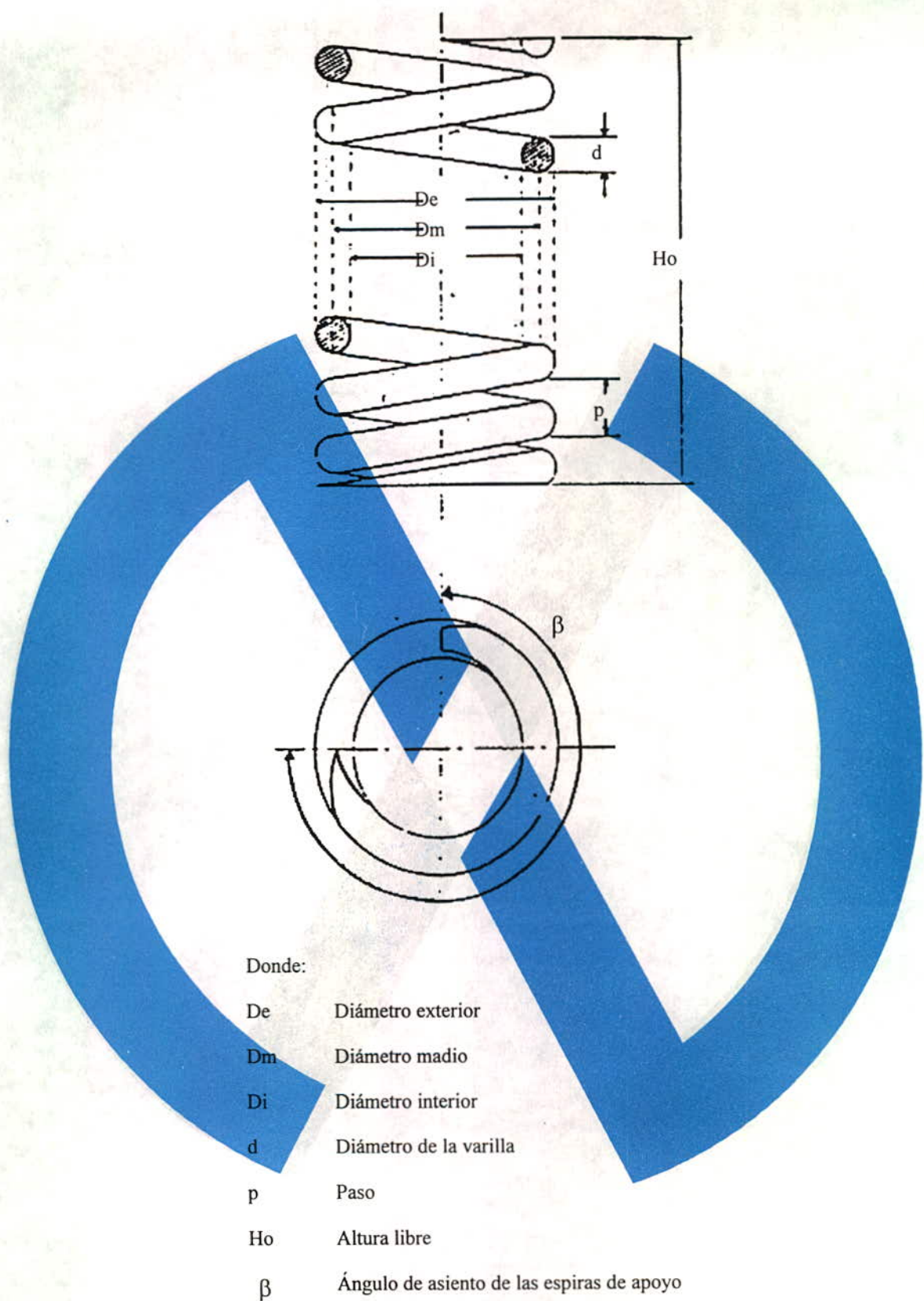
Figura 1a. Resorte de constante elástica fija
