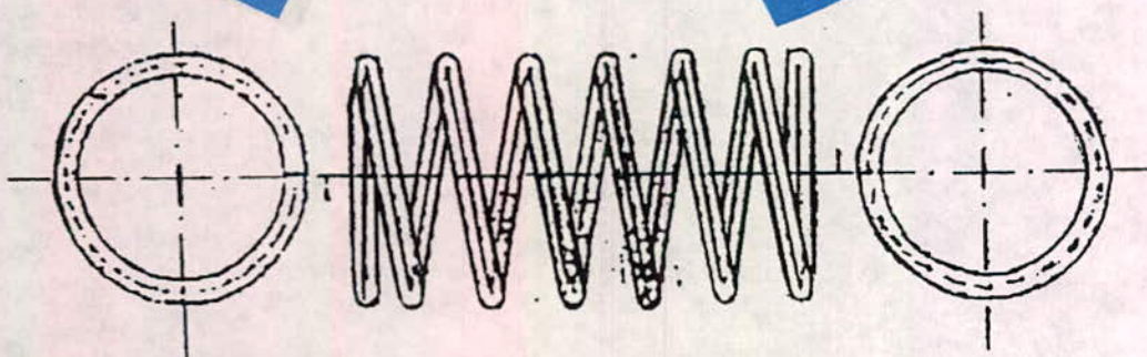
Figura 3b. Dos terminales planos sin despalmado
