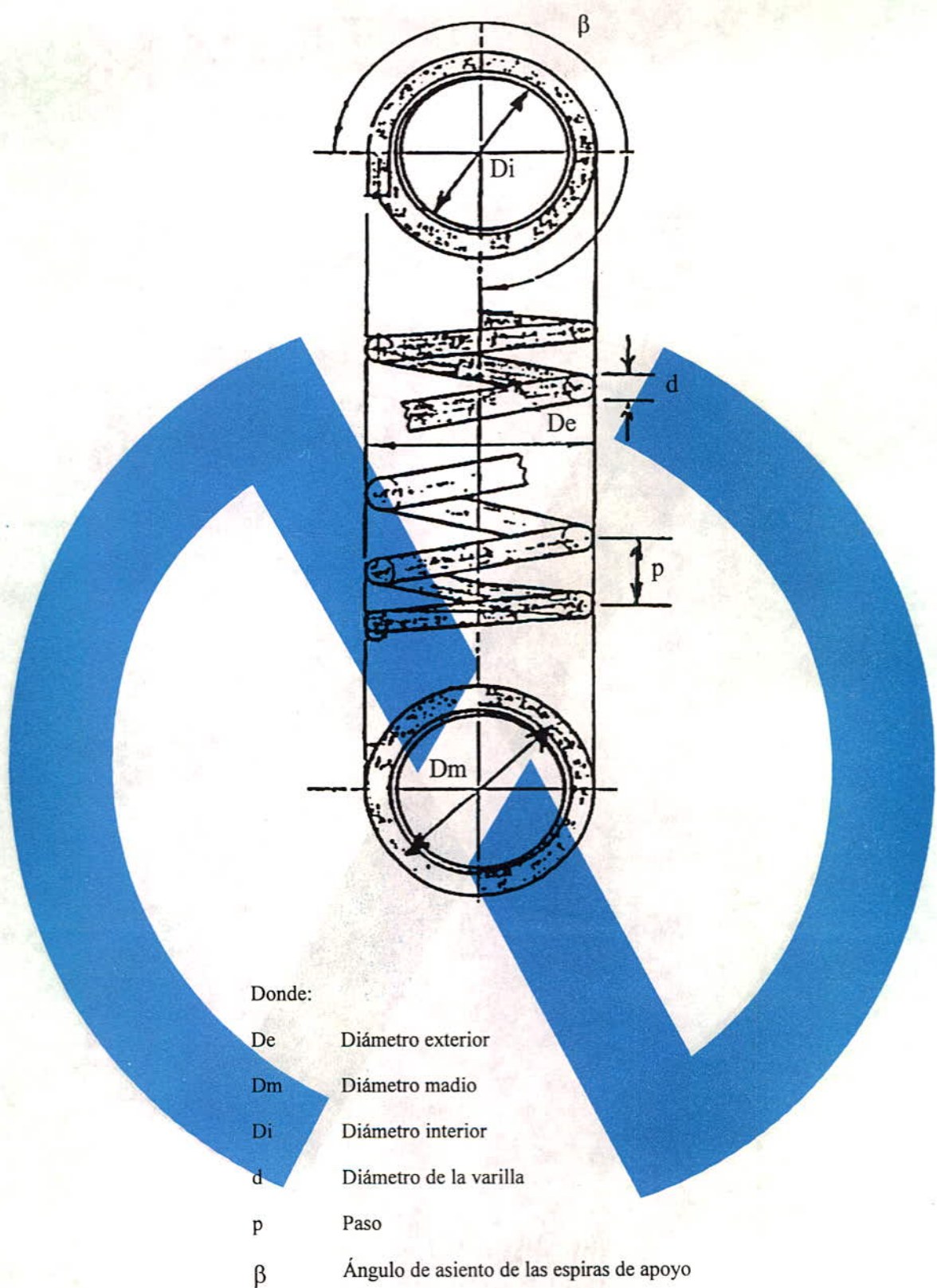
Figura 1c. Resorte de constante elástica variable
