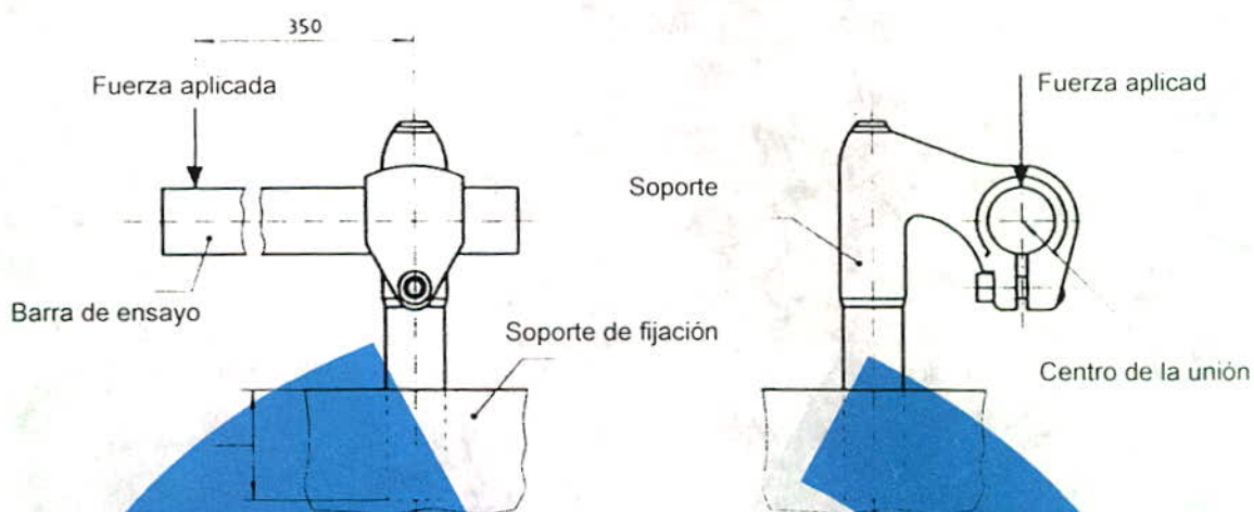
Figura 15. Ensayo de torque en el soporte del manubrio
