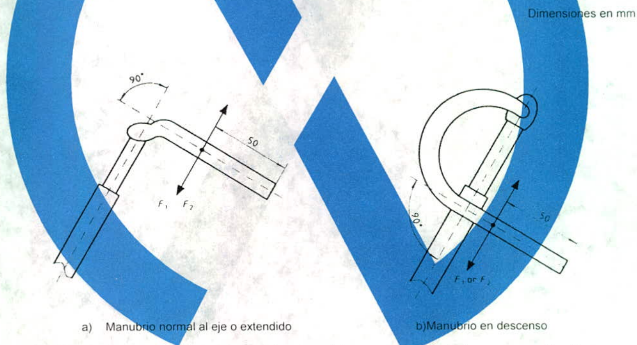
Figura 19. Orientación de los manubrios ajustables y posiciones de las cargas aplicadas
