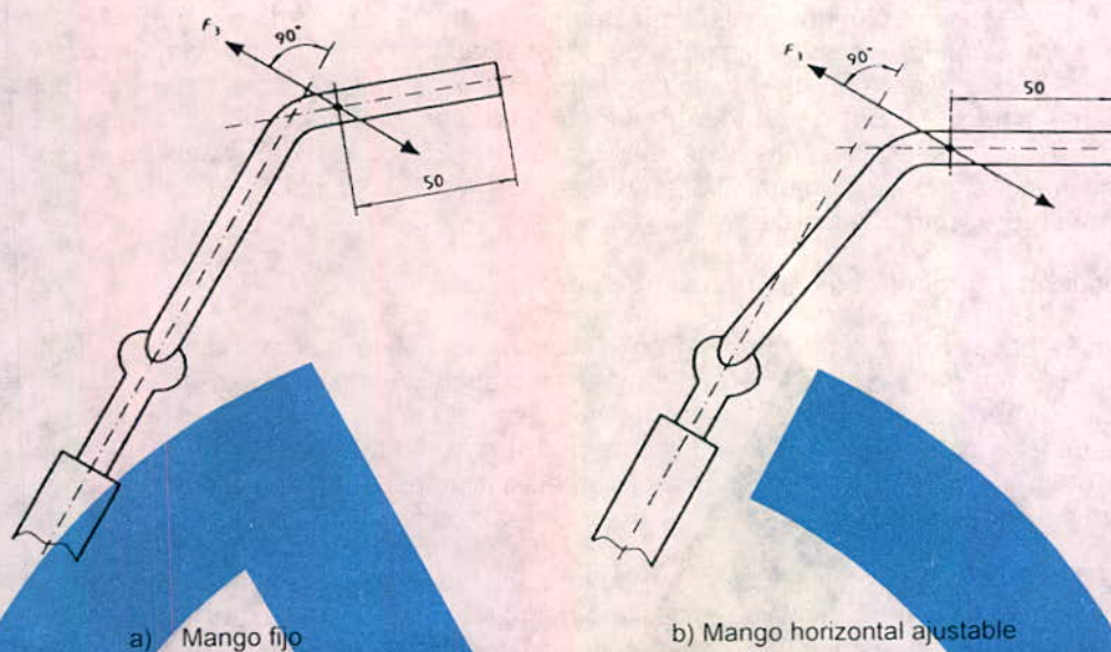
Figura 20 Manubrios de gran altura; orientación del manubrio ajustable y posiciones y direcciones de las cargas aplicadas
