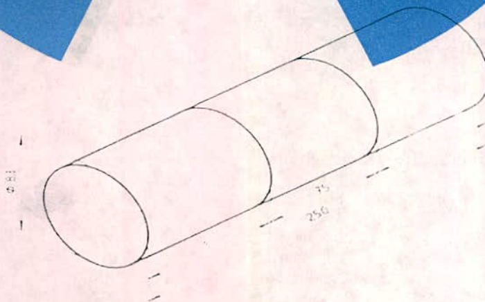
Figura 1. Cilindro de ensayo para determinar la prominencia superficial
