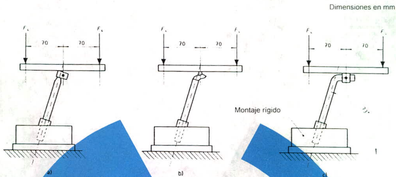
Figura 31. Disposiciones típicas de diferentes tipos de soporte de sillín para la primera etapa del ensayo (el ángulo de 73° se aplica para todos)
