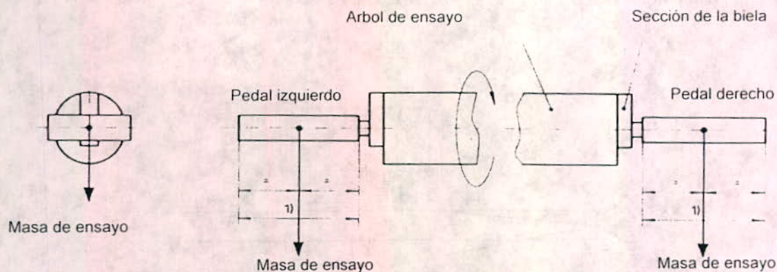
Figura 27. Ensayo dinámico de durabilidad del pedal
