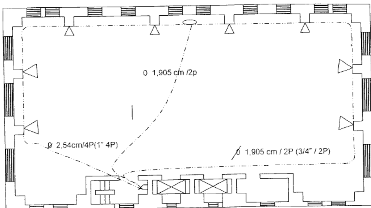
Figura 17 - Distribución típica en una planta sin división alguna
