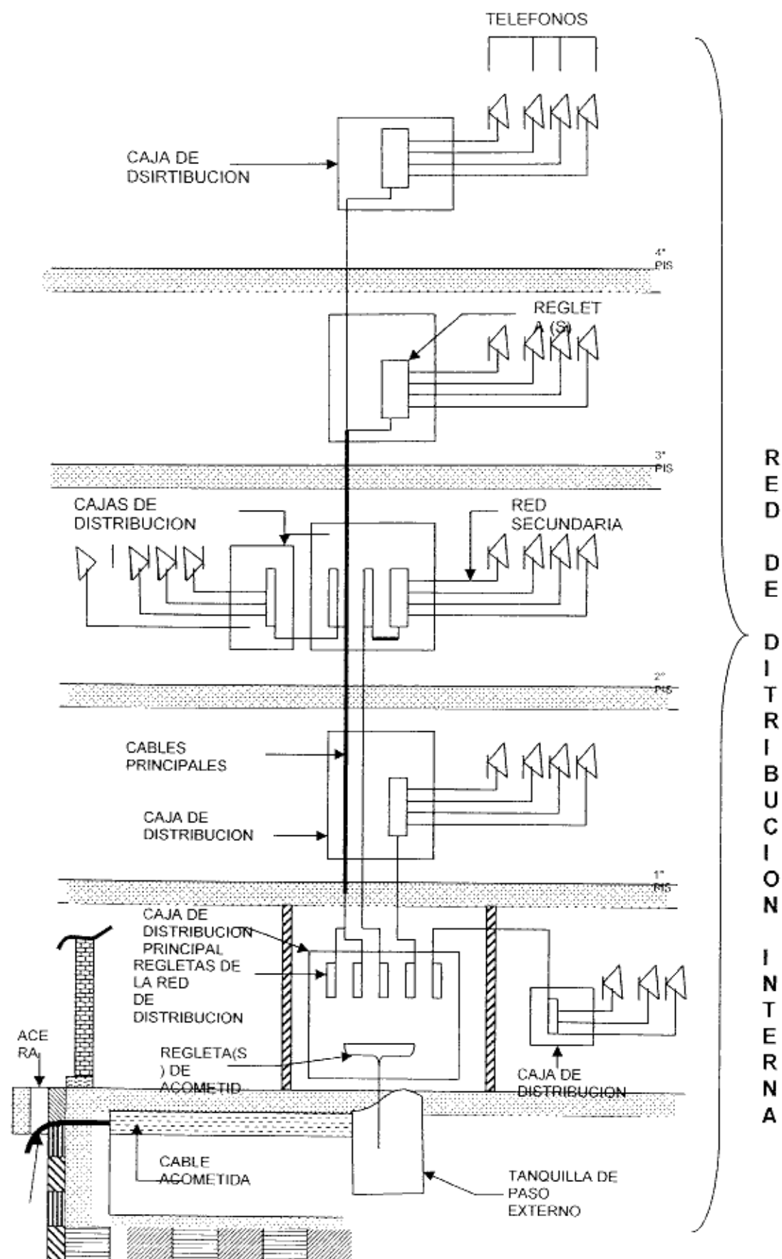
Figura 1- Esquema de la Instalación Telefónica de un Edificio
