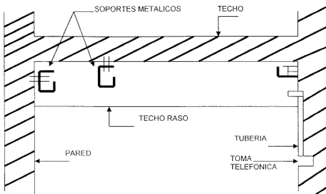
Figura 20 - Ubicación de los soportes metálicos
