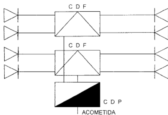
Figura 3 - Sistema de distribución radial simple
