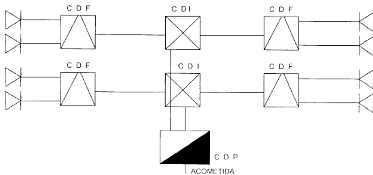
Figura 4 - Sistema de distribución radial complejo
