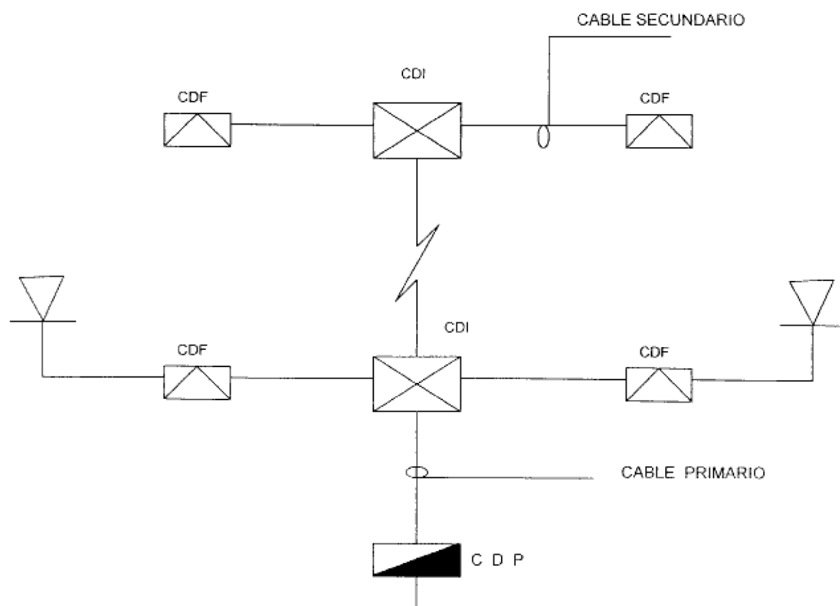
Figura 12 - Clasificación De Cables
