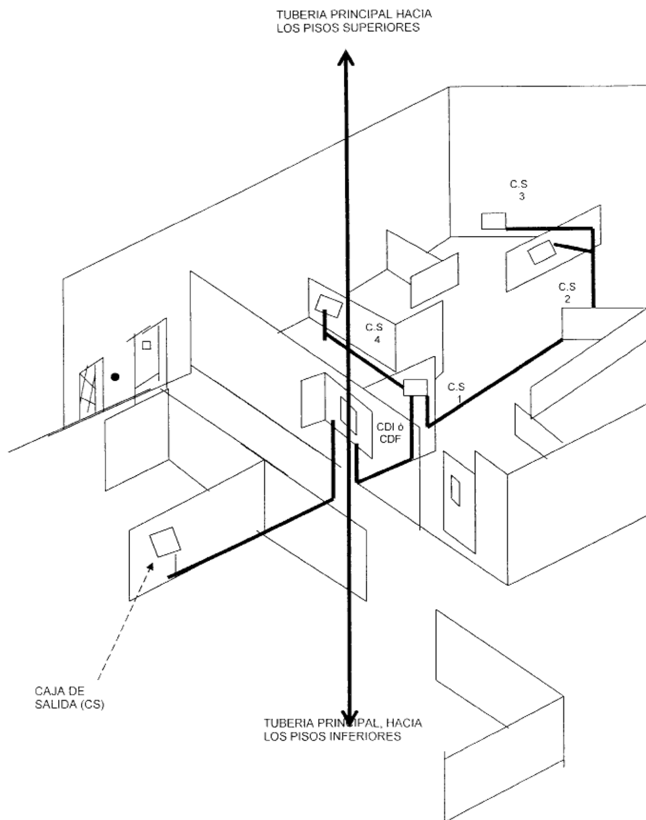
Figura 15 - Distribución radial para edificios residenciales
