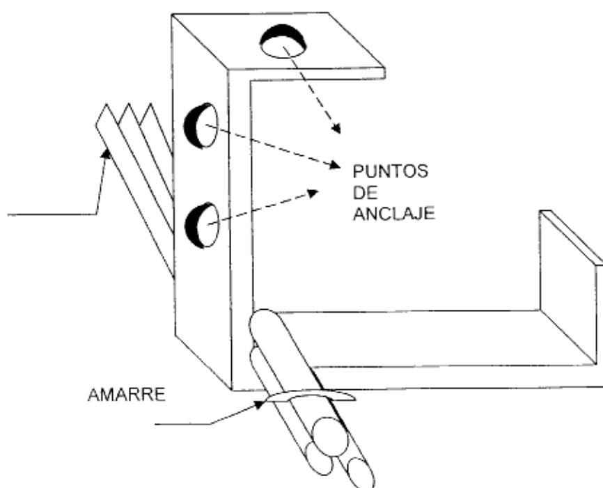
Figura 18 - Soporte Metálico
