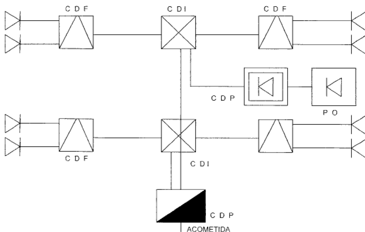
Figura 5 - Sistema de distribución radial complejo con una central privada para dar servicio a todo el edificio.
