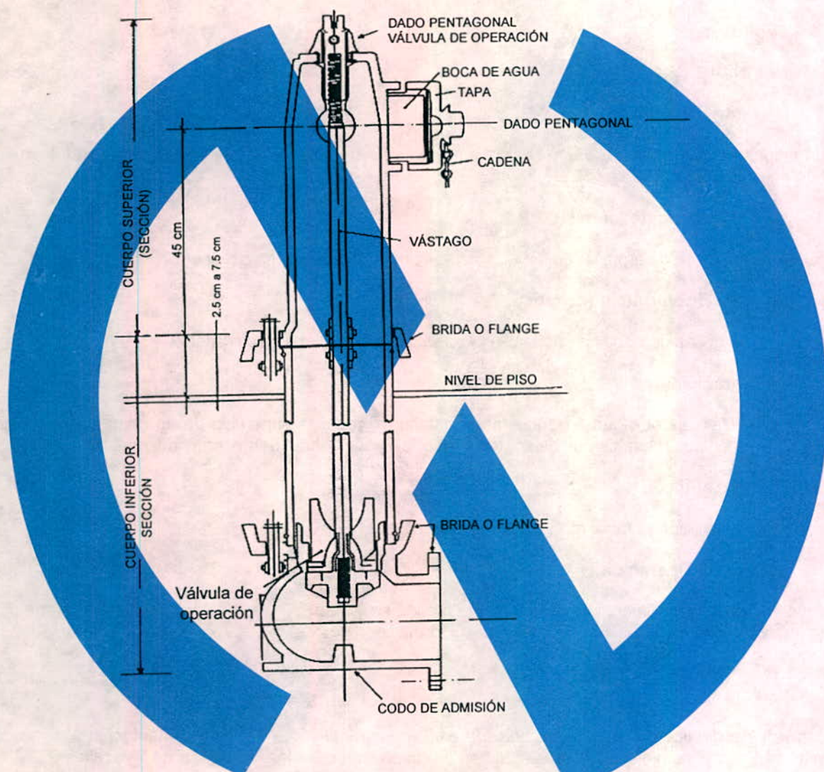
Figura 1 - Dibujo esquemático de un hidrante de poste, con válvula de operación al pie del hidrante
