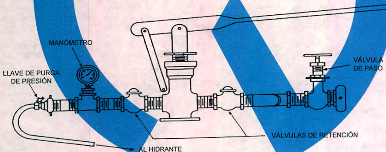
Figura 12. Bomba manual para prueba hidrostática
