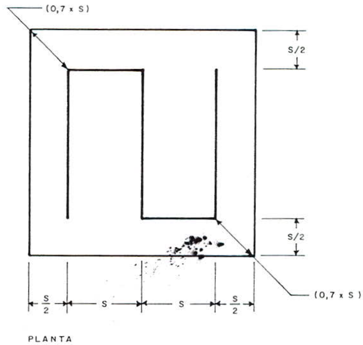
FIG. 5 DETECTORES LINEALES
