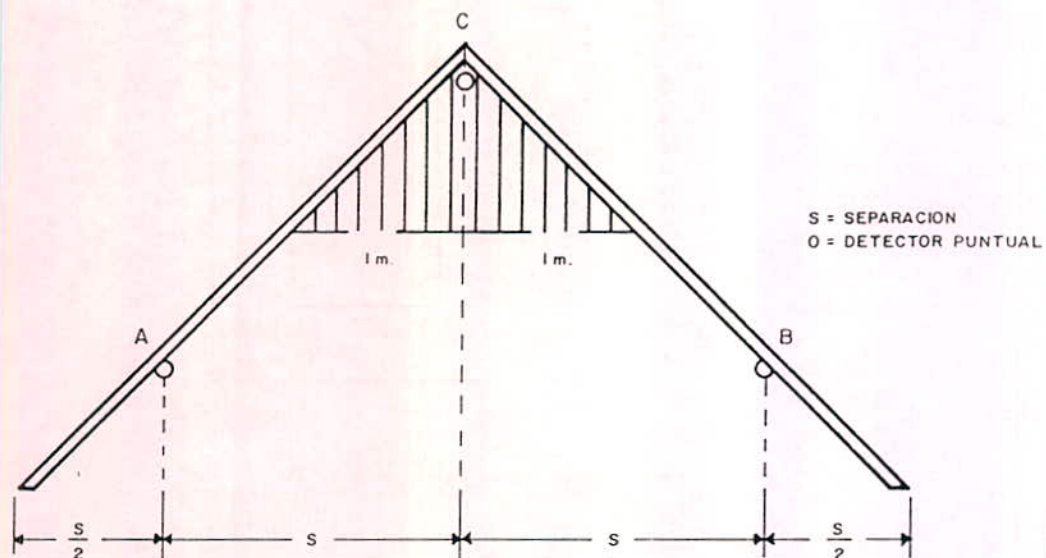
FIG. 7 CORTE ESQUEMATICO
