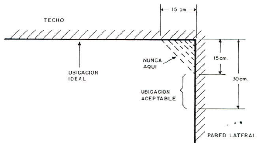
FIG. 1 UBICACION DE DETECTORES DE CALOR
